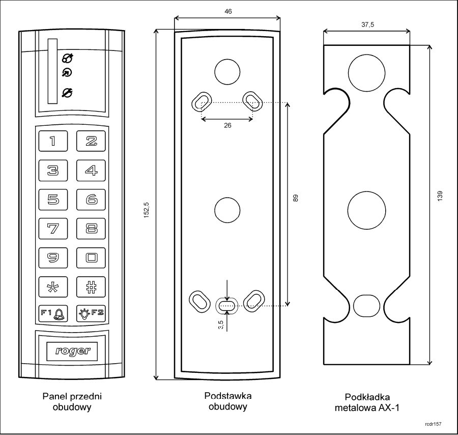
Rys.1 Widok ogólny podkładki AX-1
